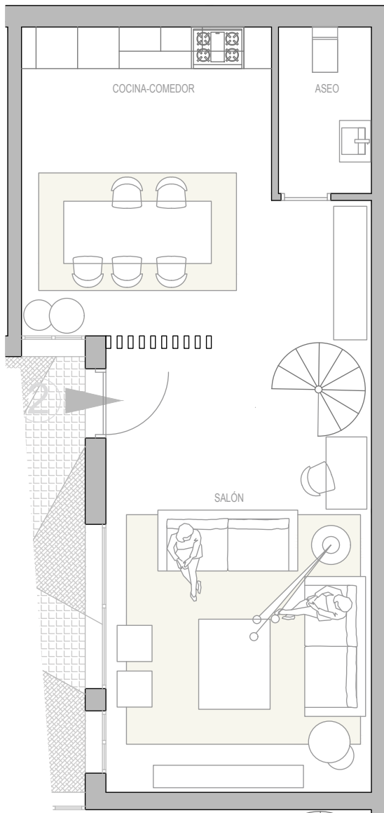
PLANTA BAJA
