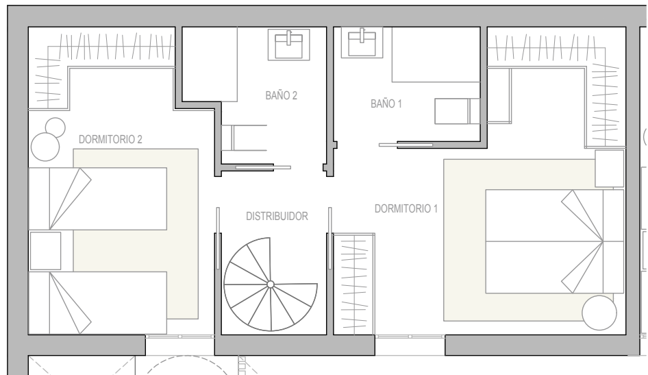
PLANTA ALTA
