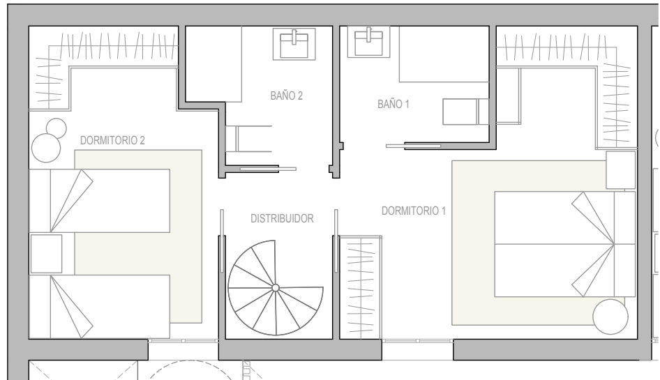
PLANTA ALTA
